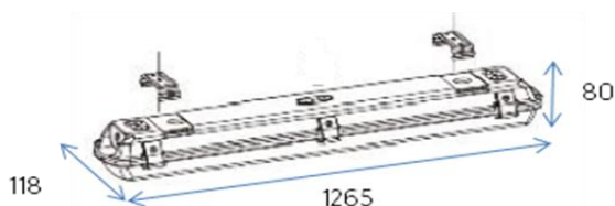
Schéma Dimensionnel Luminaire
